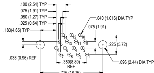
15 PIN MWDM-15PCBS
