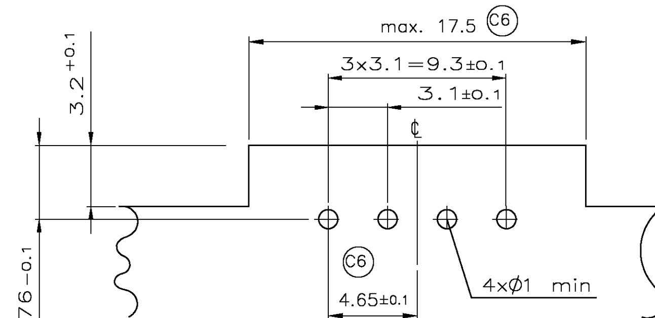
Leiterplattenlayout PCB-LAYOUT
