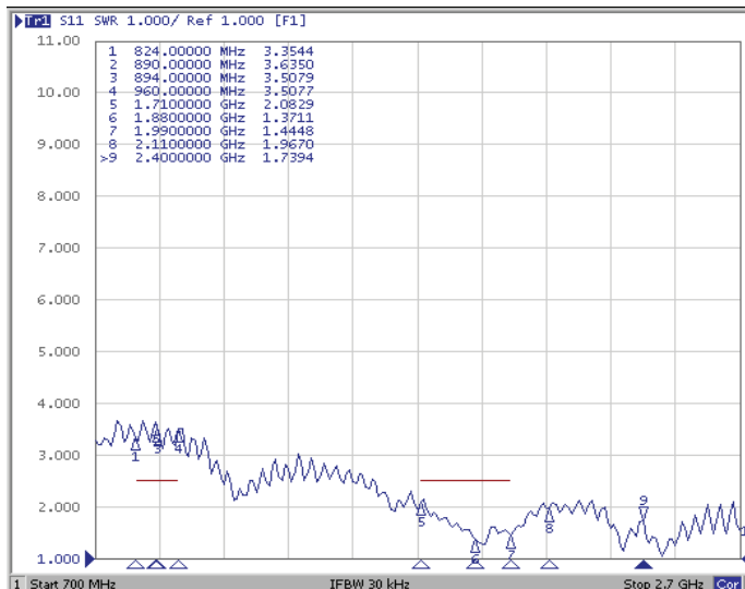
VSWR (S11)
