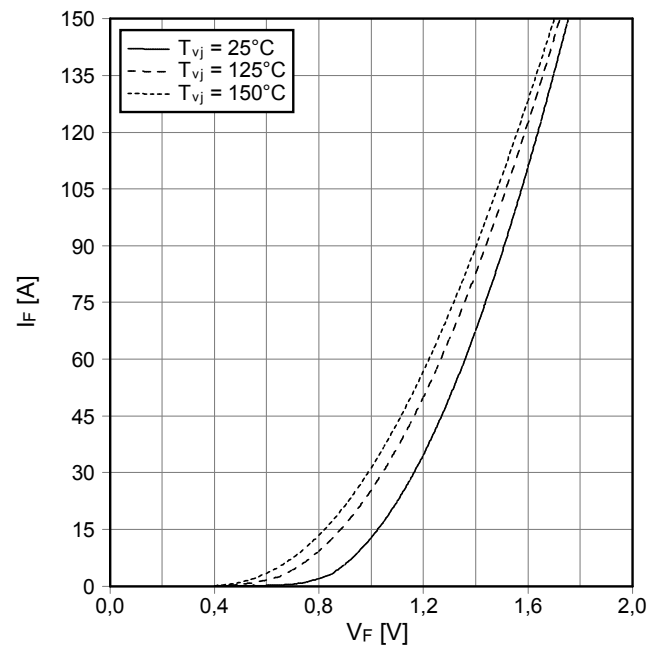
Durchlasskennlinie der Diode D5 - D6 forward characteristic of Diode D5 - D6 I_F = f(V_F)
