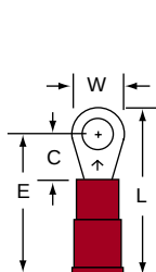
MNG18-6R/S Stud Size 6 Wire Range 22-18
