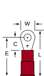
MNG18-4R/S Stud Size 4 Wire Range 22-18
