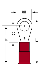
MNG18-10R/L Stud Size 10 Wire Range 22-18
