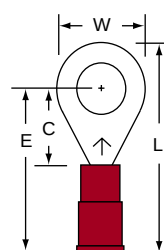
MNG18-14R/S Stud Size 1/4 Wire Range 22-18
