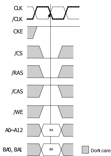
Figure12 : Active command
