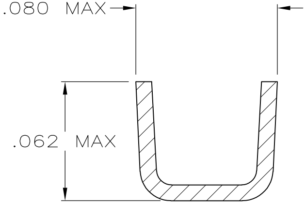
SECTION A-A SCALE 20:1
