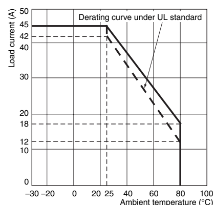
G3PB-245B-3-VD G3PB-245B-2-VD
