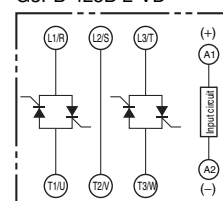
G3PB-425B-2-VD
