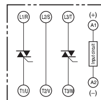
G3PB-215B-2-VD
