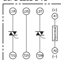
G3PB-225B-2-VD
