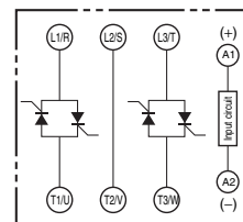
G3PB-4□5B-2H-VD
