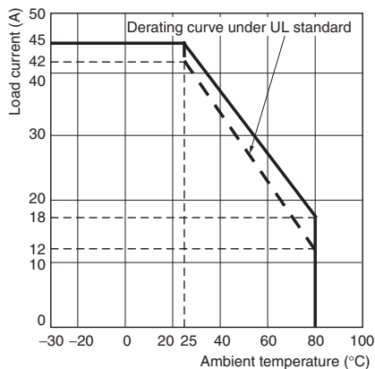
G3PB-445B-3-VD G3PB-445B-2-VD
