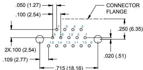
15 SOCKET
