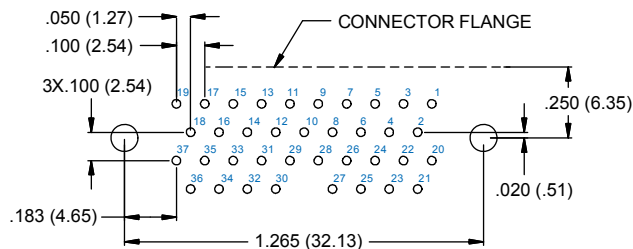
37 SOCKET
