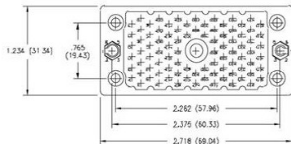
120 PIN RECEPTACLE
