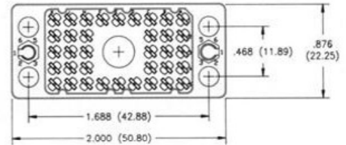
36 PIN RECEPTACLE
