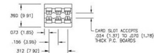
6 CONTACT CENTRE MODULE
