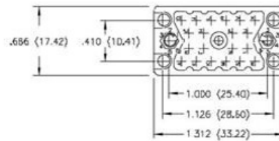
20 PIN RECEPTACLE
