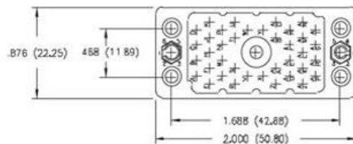
38 PIN RECEPTACLE
