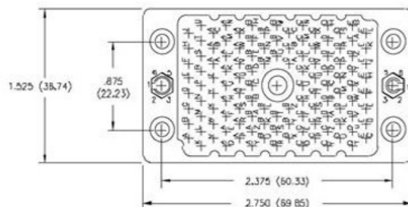
120 PIN RECEPTACLE
