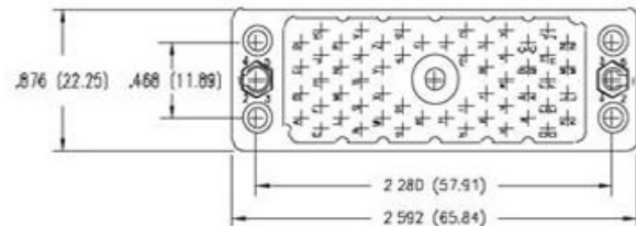
90 PIN RECEPTACLE
