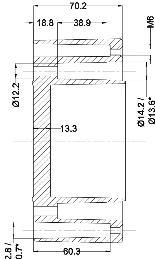
SECTION A-A
