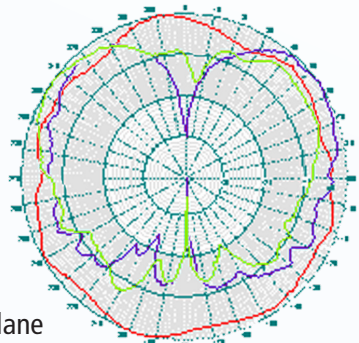
5.15 GHz
