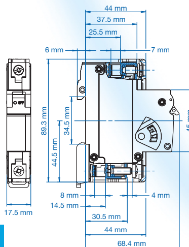
Dimensions N63UM, FxaxxUM.
