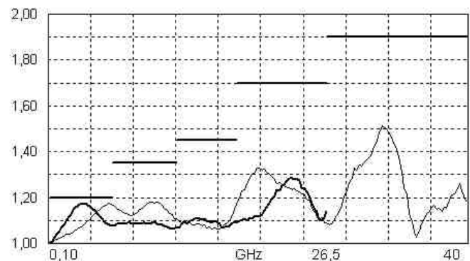
V.S.W.R.
