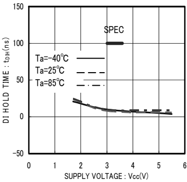
Fig.16 DI Hold time t_{DIH}
