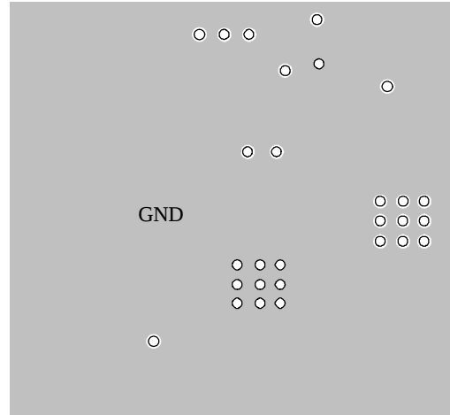
Inner1 Layer
