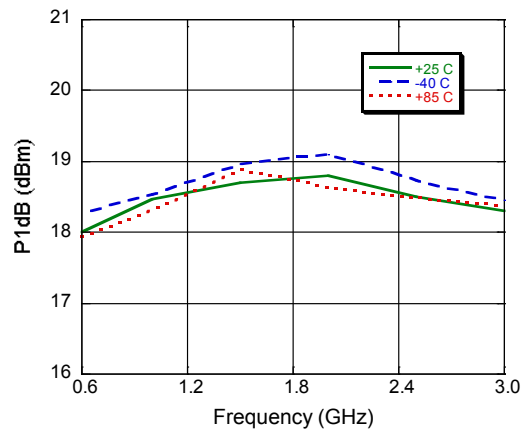
P1dB
