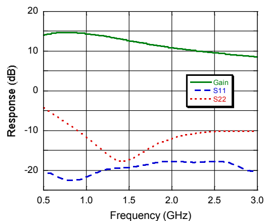
S-Parameters
