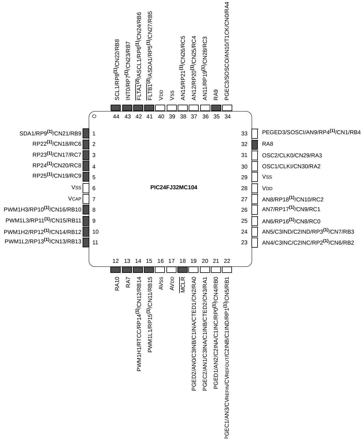
44-Pin TQFP
