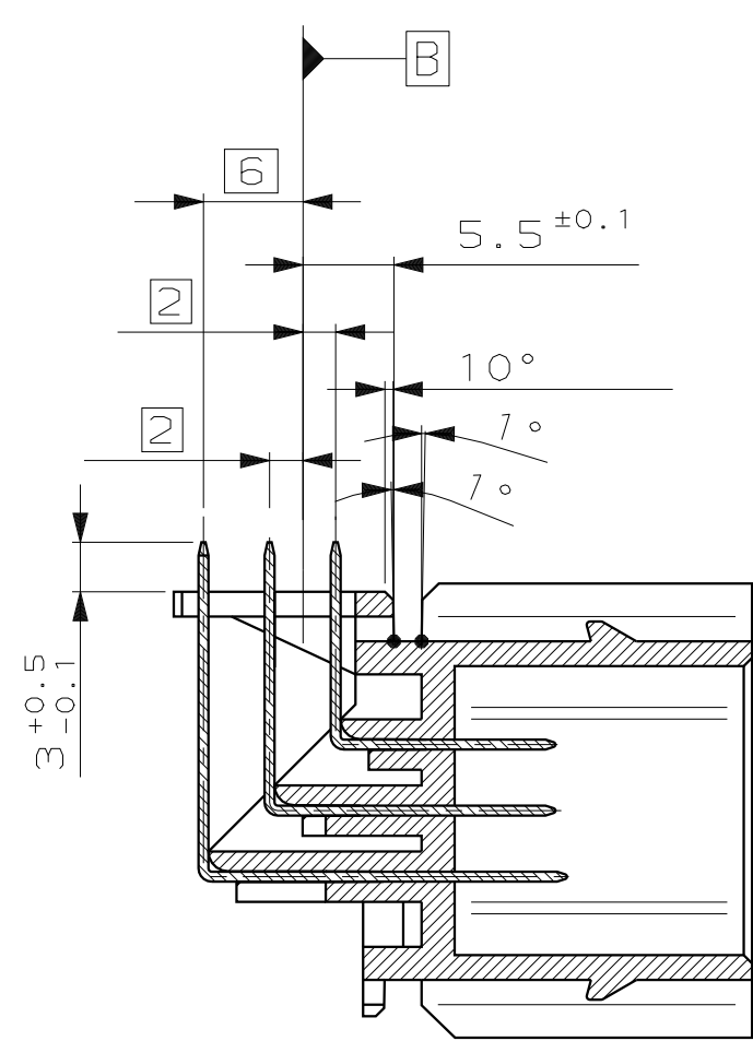
Schnitt A-A
