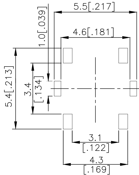
P.C.B. LAYOUT
