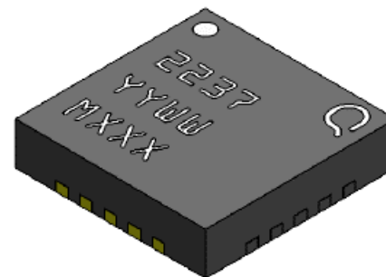
QFN 4x4 mm 20L
