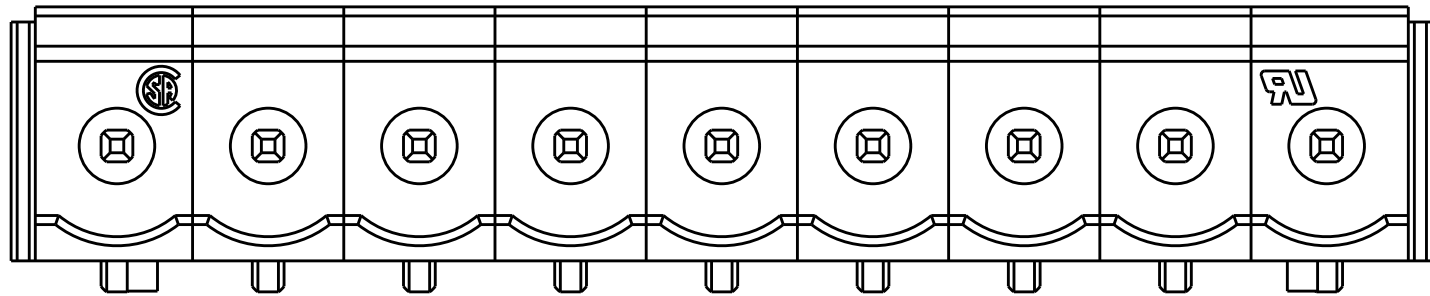
9 POLES: 2305908-9
