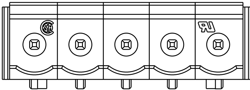
5 POLES: 2305908-5
