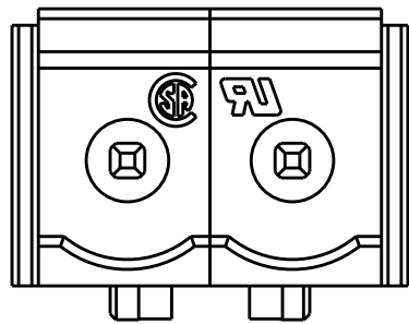
2 POLES: 2305908-2
