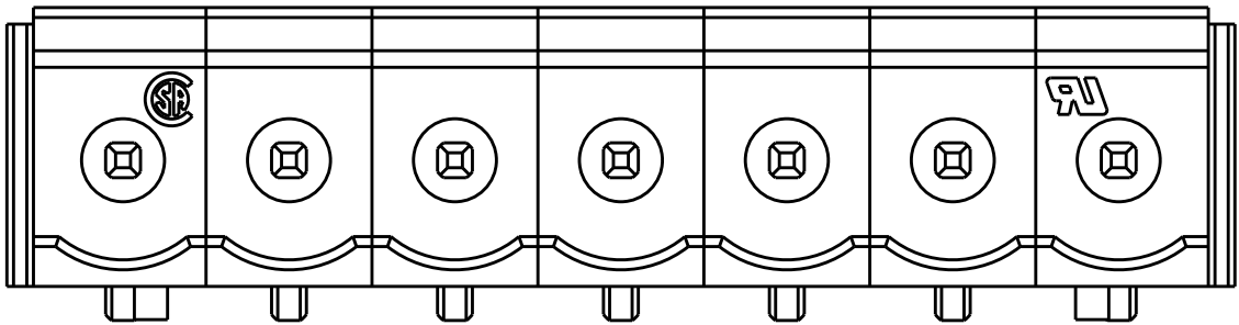
7 POLES: 2305908-7
