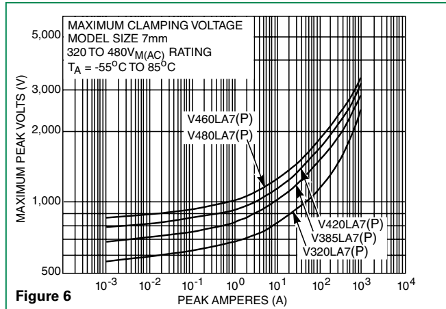
V320LA7(P) - V480LA7(P)
