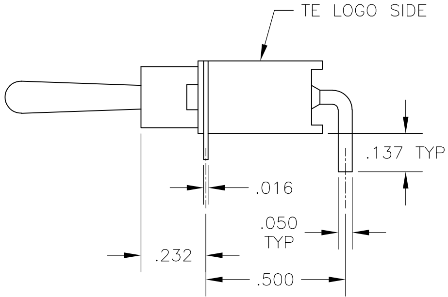
D1 BUSHING
