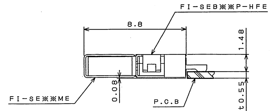
COUNTERPART CONNECTOR 相手側コネクタ
