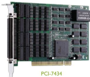
PCI-7434
