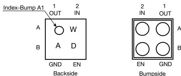
Fig. 2 - WCSP 2 x 2 Package
