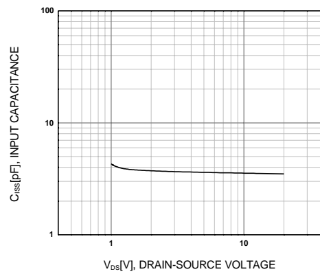
Figure 6. C_{ISS} - V_{DS}
